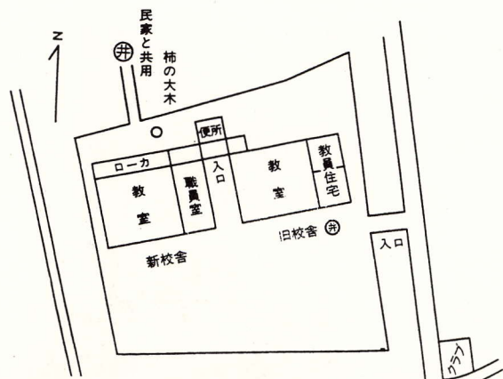
岡上分教場 平面図 昭和5年以後
